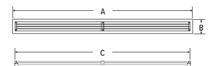
VUE AVANT
